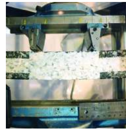
Δοκιμαστική διάταξη
